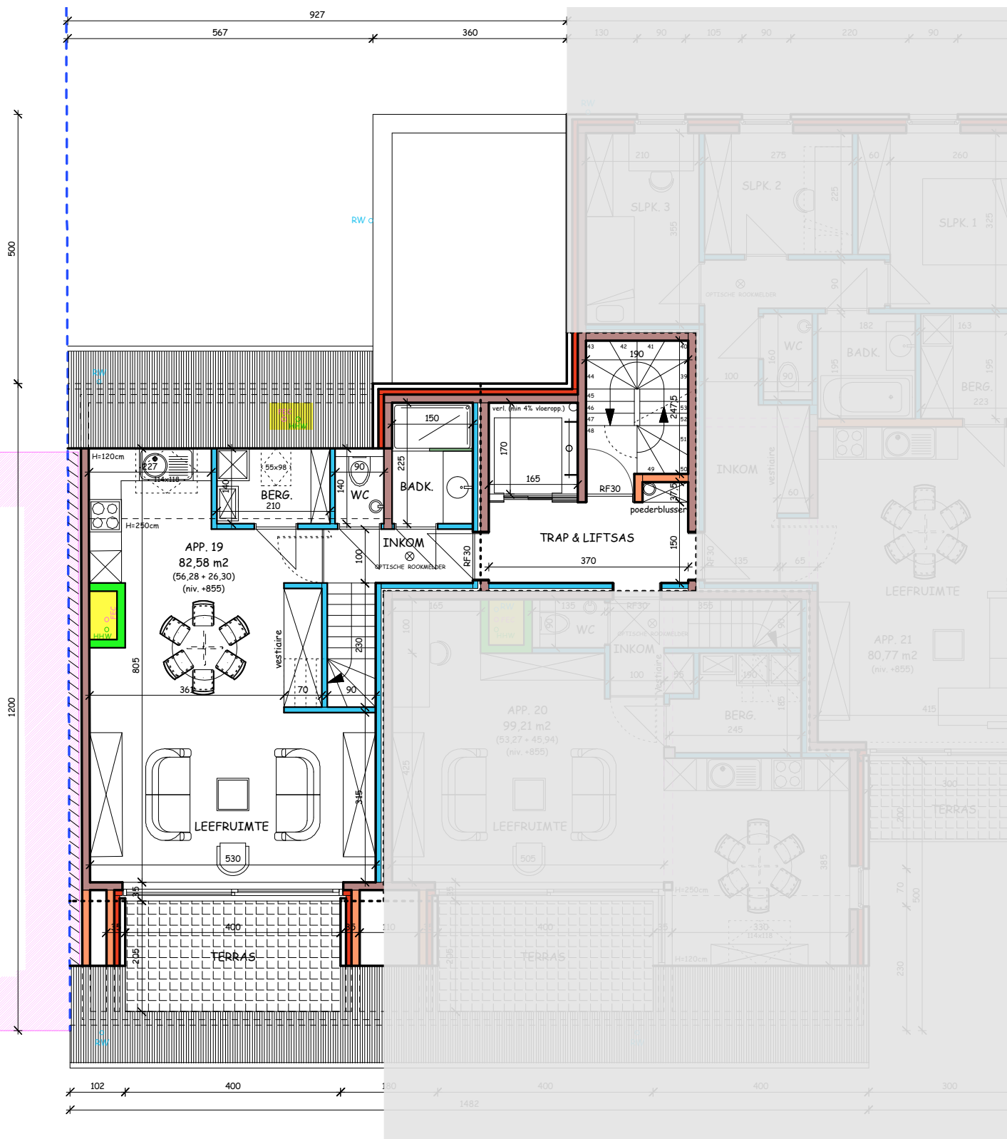
APPARTEMENT 19a - VERDIEPING 3 (schaal 1/100)
